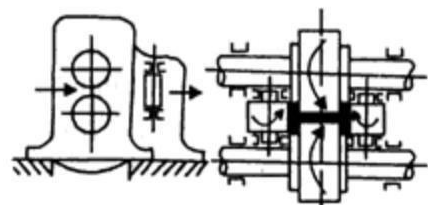
(f) Universal roll mill.
