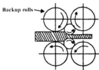
(d) Cluster rolling mill.
